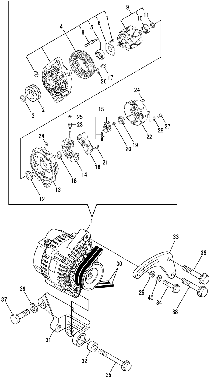
Fig.58. GENERATOR
