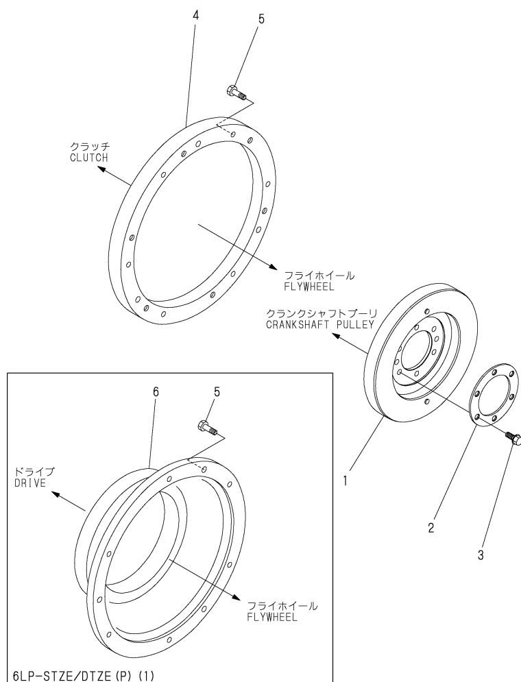
Fig. 22 ダンパ DAMPER
