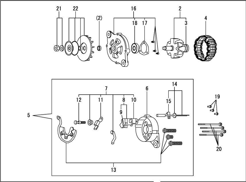
Fig.38. GENERATOR(12V-80A)
