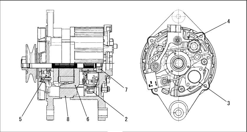
Fig.53. (33A)GENERATOR(EARTH FLOATYPE)(BOSCH)
