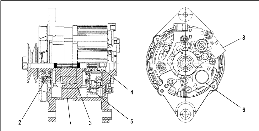
Fig.52. (32A)GENERATOR(BOSCH)
