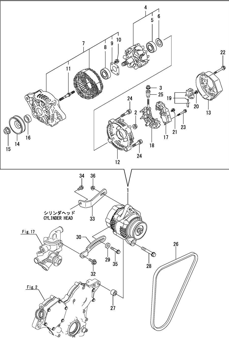
Fig.32. GENERATOR
